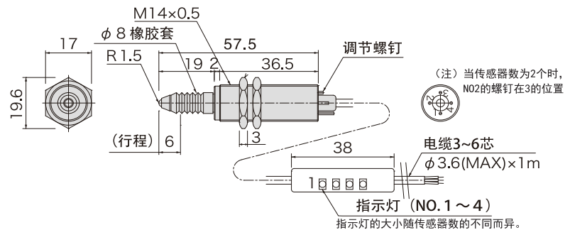
尺寸图
